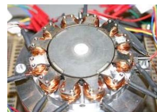
図2 試作したベアリングレスモータ。重症心疾患患者の血液循環を補助する体内植込形補助人工心臓への応用を見据えている。モータ定格出力は10Wである。
